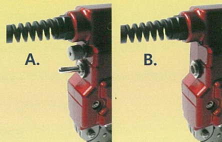
A. AC / DC Type B. AC only
